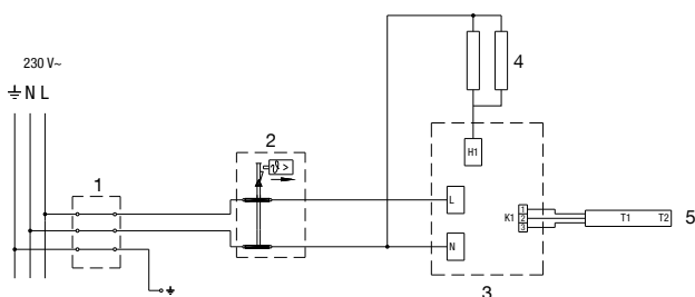
Obr. 6: Schéma elektrického pripojenia
