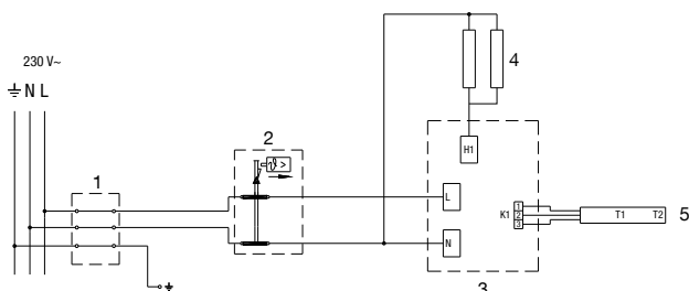
Obr. 6: Schéma elektrického připojení
