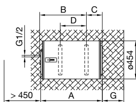
Obr. 2: Vodorovná inštalácia na stenu
