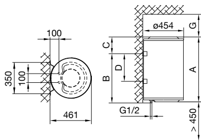
Obr. 1: Zvislá montáž na stenu
